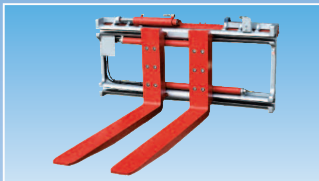
RZV-GS, separate sideshift, geschroefde vorken
