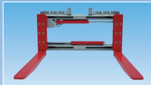
RZV-G, ventielgestuurde sideshift, geschroefde vorken
