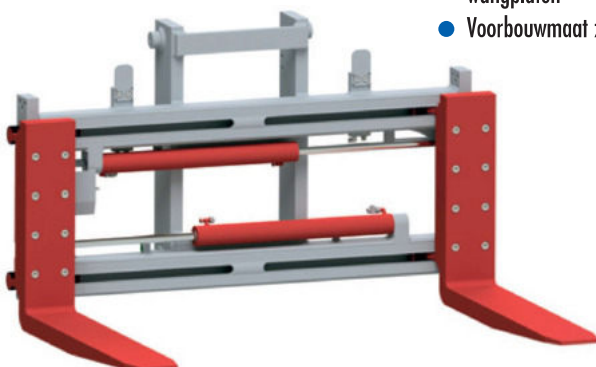
Optie: beschermbeugel
