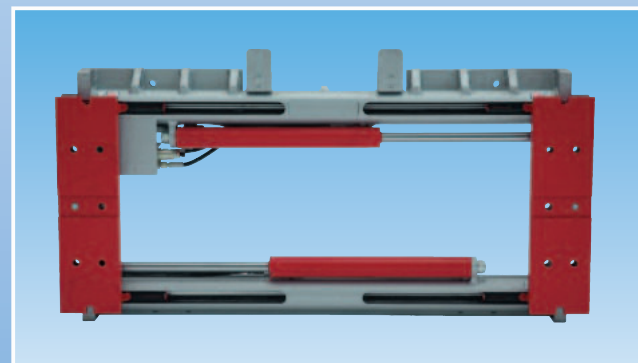
RZV, ventielgestuurde sideshift, voor ISO / FEM vorken
